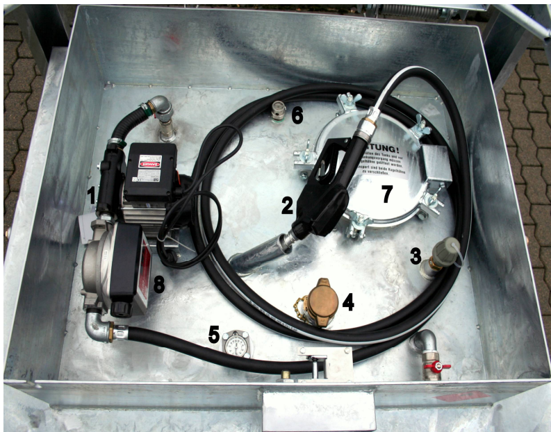
Armaturenordnung
